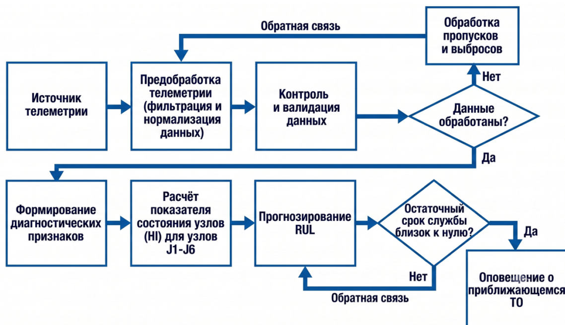
Рисунок 14 - алгоритм прогнозирования остаточного ресурса
